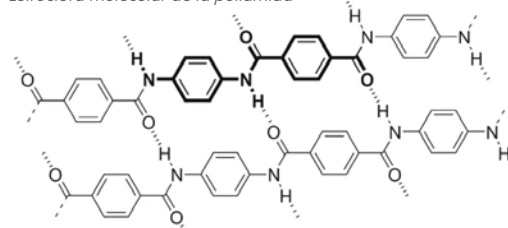
Estructura molecular de la poliamida
